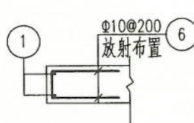
洞口附加筋
