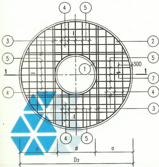
YB-I-1~3配筋图
